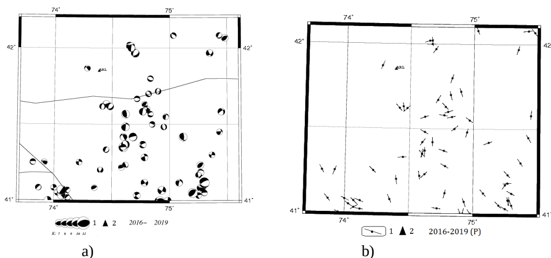
Рисунок 7. Карта-схема: а) механизм очагов землетрясений (1 - механизмы, 2 - сеймостанция) и б) ориентации осей напряжения сжатия (1 - направление азимутов сжатия, 2 - сеймостанция) в очагах землетрясений в районе сеймостанции «Арал» (ARL) за 2016-2019 гг. ( \varphi = 41^{\circ}00' - 42^{\circ}06' и \lambda = 73^{\circ}45' - 75^{\circ}30' ).
