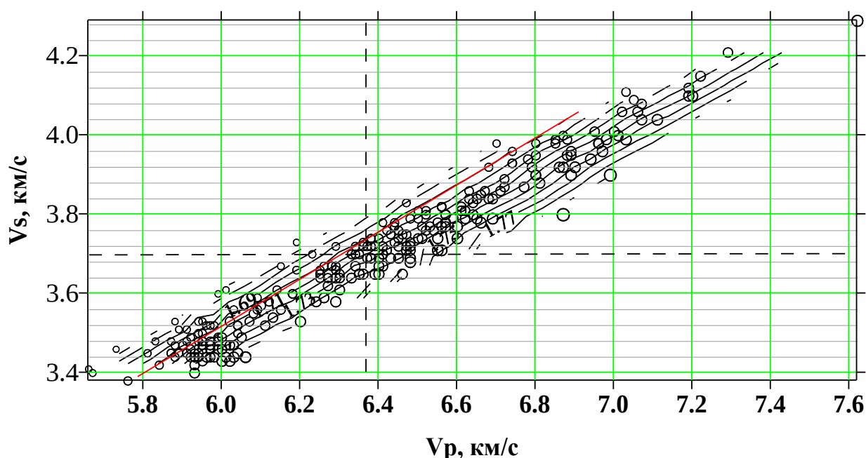
Рисунок 13. Соотношение между V_p , V_s , V_p/V_s взрывов в квадрате \varphi=41.79^\circ - 41.87^\circ , \lambda=78.17^\circ - 78.28^\circ Центрального карьера Кумторского месторождения. Кружочками обозначены наблюденные значения V_p/V_s . Значение V_p/V_s = 1.72 выделено диагональной красной линией. Выше этой линии выделяются параллельные линии, где кружочки имеют малые значения V_p/V_s < 1.72 , а ниже данной линии отмечаются параллельные линии, где кружочки имеют большие значения V_p/V_s > 1.72
