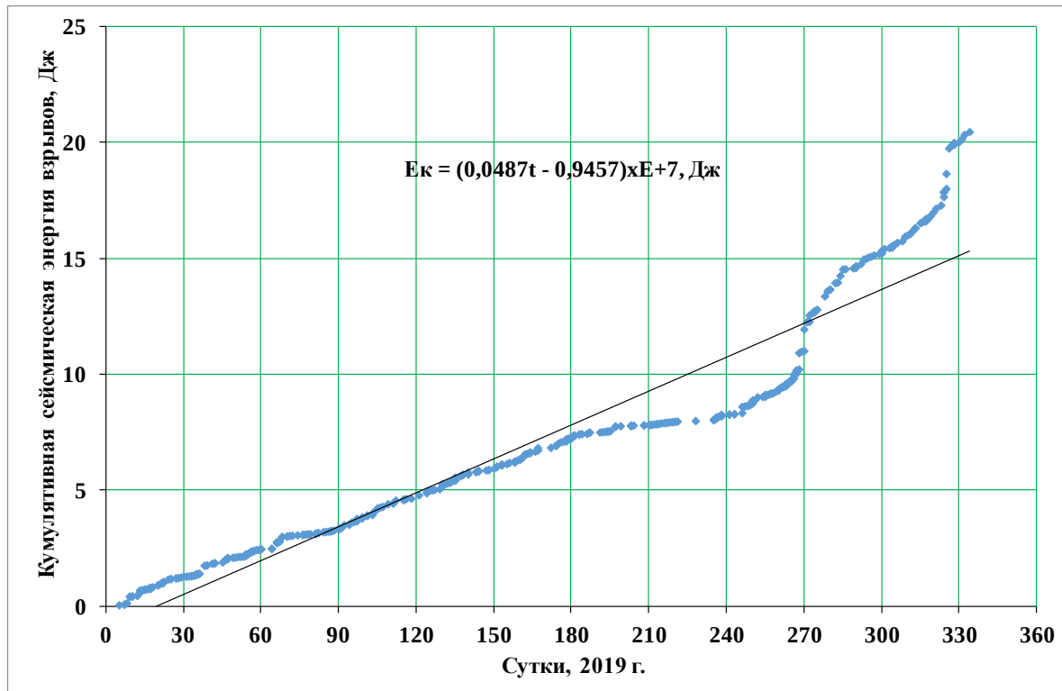
Рисунок 4. Кумулятивная сейсмическая энергия, высвобожденная при взрывах в пределах карьера «Центральный» за январь-ноябрь 2019 г.
